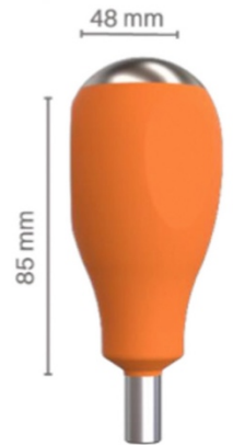
OM 14-0890 K48 Handle SS End Cap
